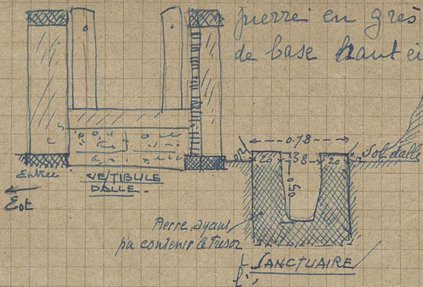
COUPE S/ VESTIBULE ET SANCTUAIRE.
