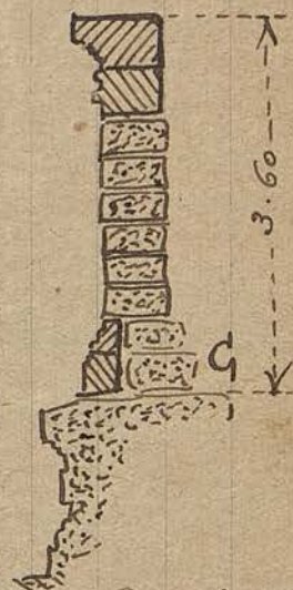
Coupe sur le mur A ci-contre
