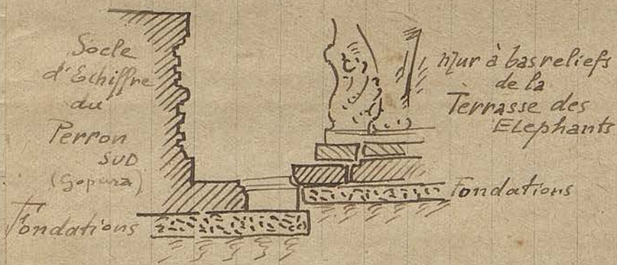
Coupe sur le Raccord Sud du Gopura E du Palais Royal avec la Terrasse des Elephants (Voir Photos 921-922)
