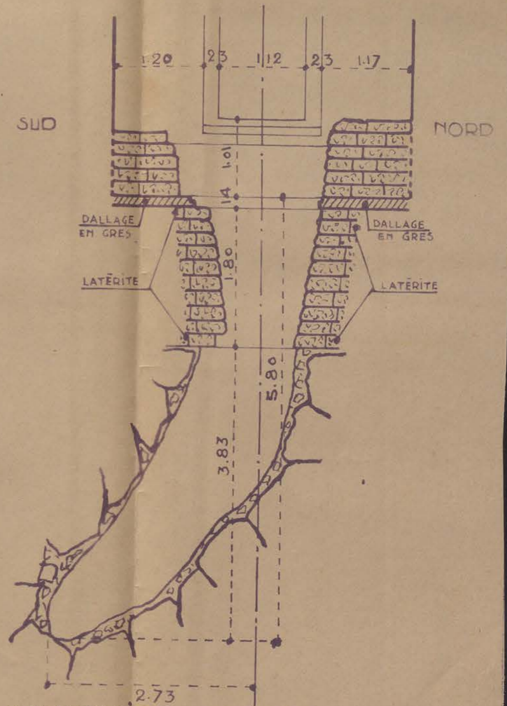
SANCTUAIRE CENTRAL COUPE NORD SUD
