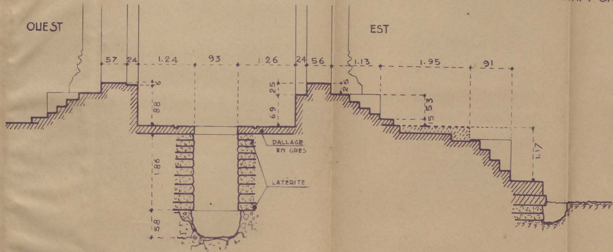
SANCTUAIRE SUD COUPE EST OUEST
