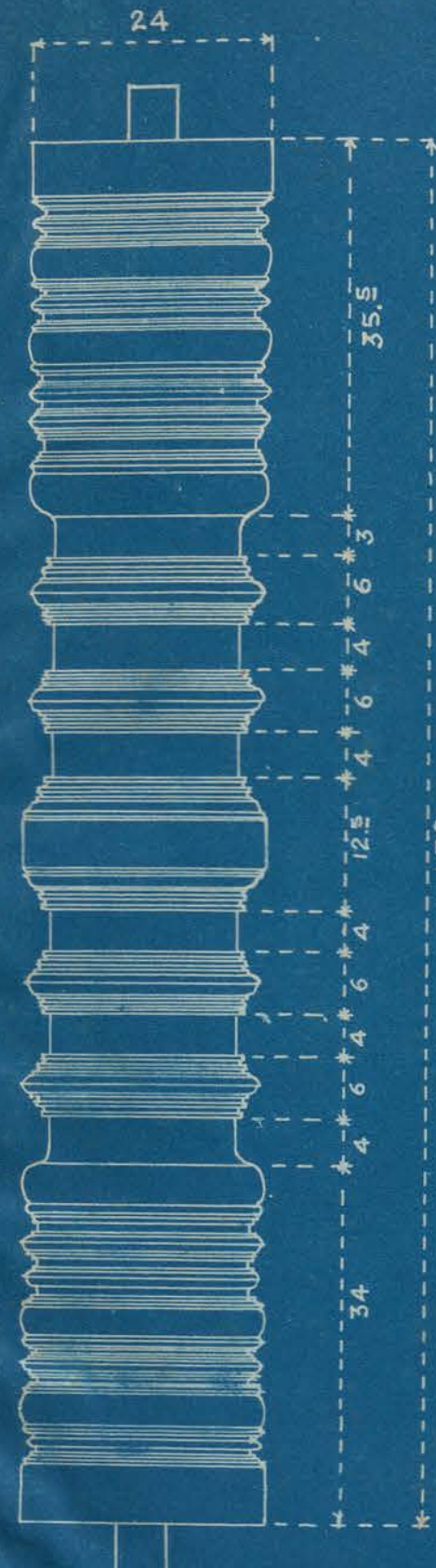
TYPE DE BALUSTRE (TROUVÉ PRÈS DU BÂTIMENT SUD H.) ECHELLE 0 m /15 P. M.
