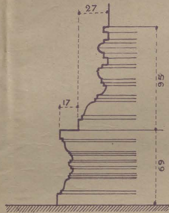
BASE DU SANCTUAIRE COUPE SUIVANT C D ECHELLE 0.05 P.M.
