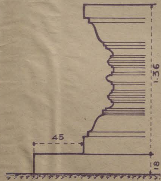
SOUBASSEMENT COUPE SUIVANT A B ECHELLE 0.05 P.M.
