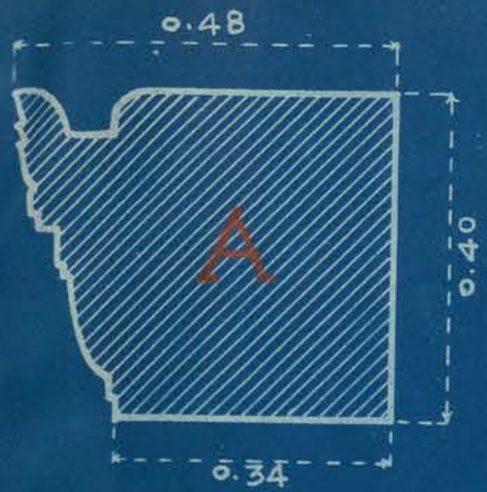
CORNICHE DU COURONNEMENT DES MURS, A LOTUS Echelle 0.10 p.m.
